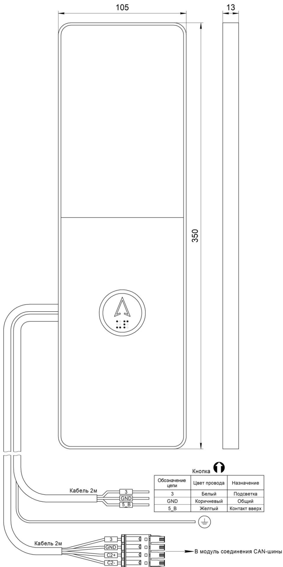
Рис.1 Внешний вид, габаритные и установочные размеры Вызывного поста МАЛАХИТ НШЕК.468381.015-20
